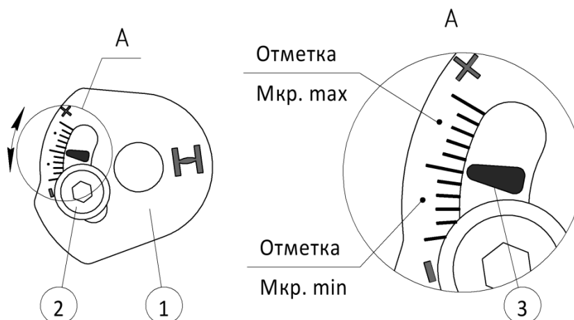
Рисунок 5 – Настройка момента выключения – закрытие.
