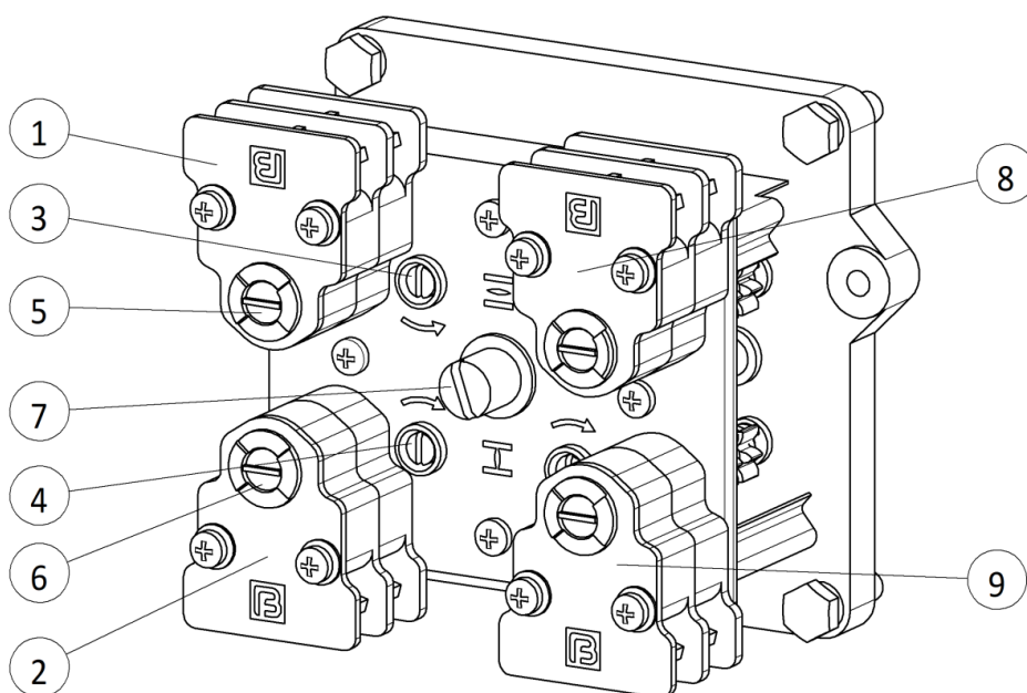
Рисунок 14 – Ограничитель хода с путевыми выключателями
