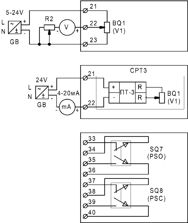
Рисунок Б.3 – Схемы подключения дополнительного оснащения привода (опции)
