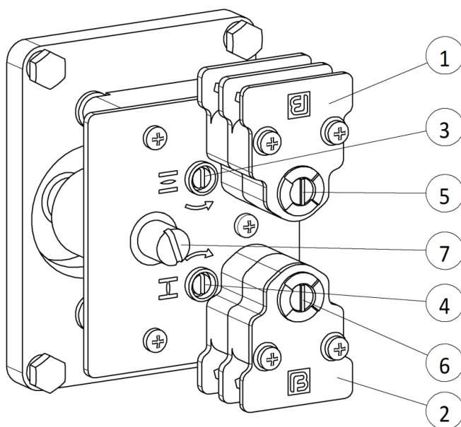
Рисунок 8 – Ограничитель хода с концевыми выключателями
