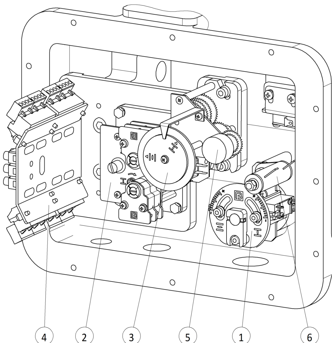
Рисунок 2 – Панель управления
