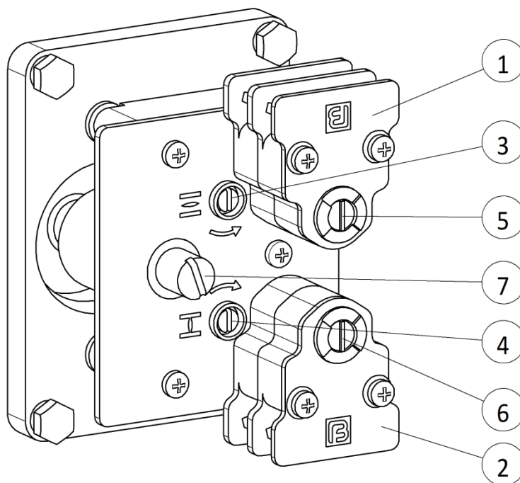
Рисунок 9 – Ограничитель хода с концевыми выключателями
