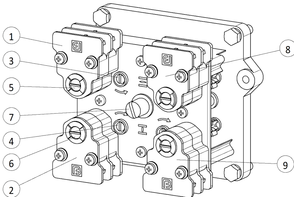
Рисунок 15 – Ограничитель хода с путевыми выключателями
