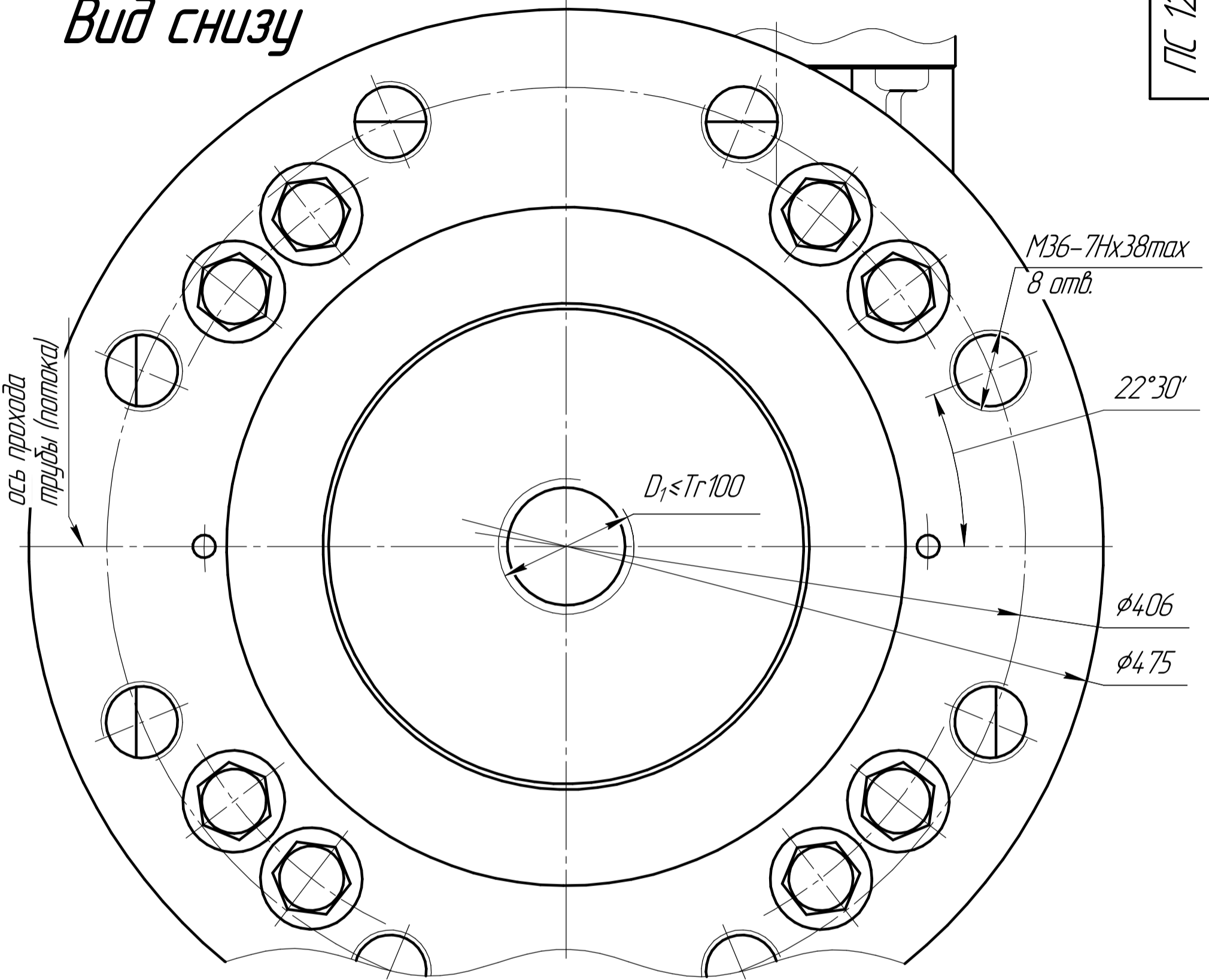
Рис. 6. Остальное см. рис. 1 F40 (Group A) по ISO 5210 (F40M (Группа А) ГОСТ Р 55510)
