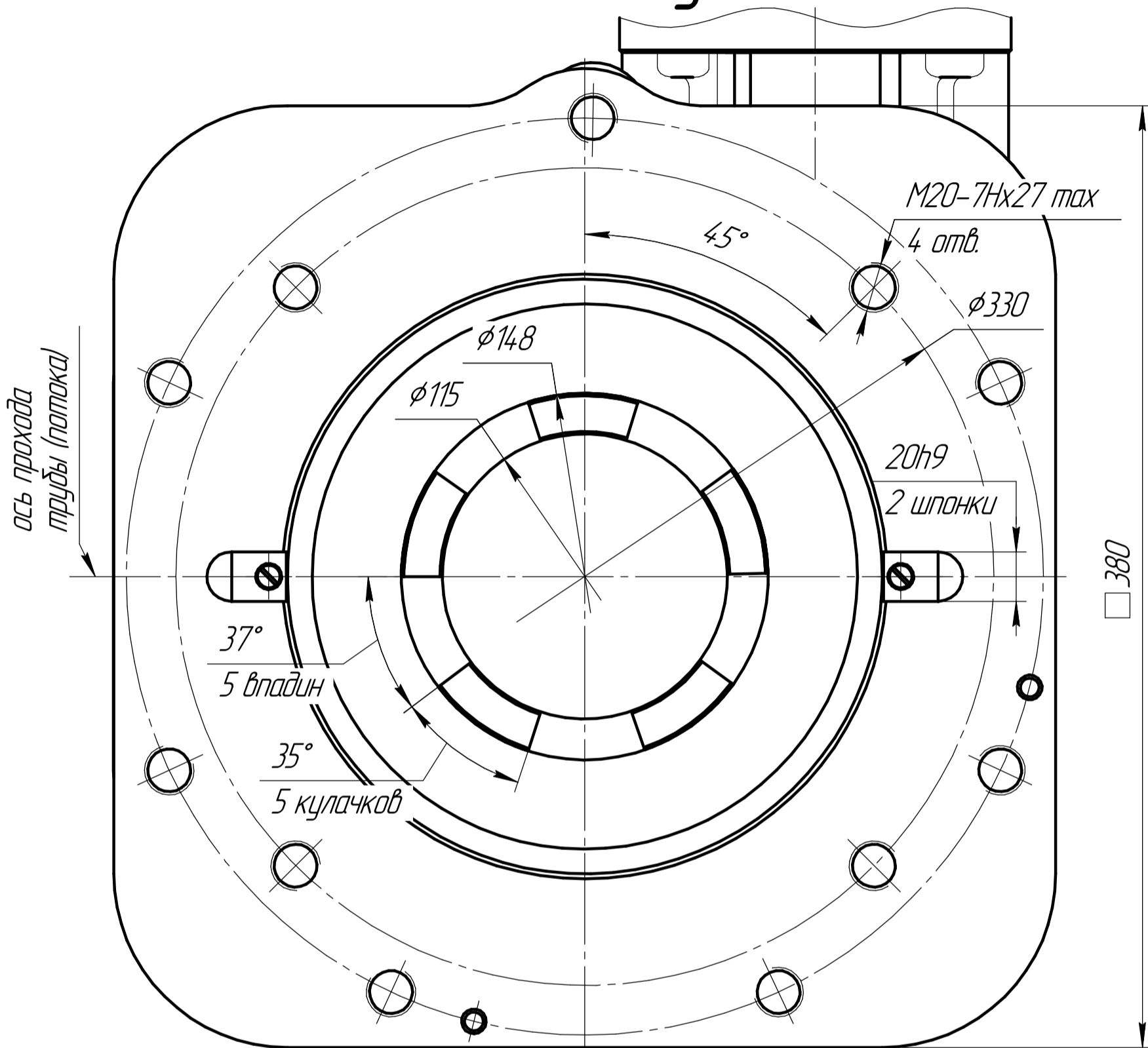
Рис. 2. Остальное см. рис. 1 Тип Г (ХХ.24) по ОСТ 26-07-763-73 Вид снизу
