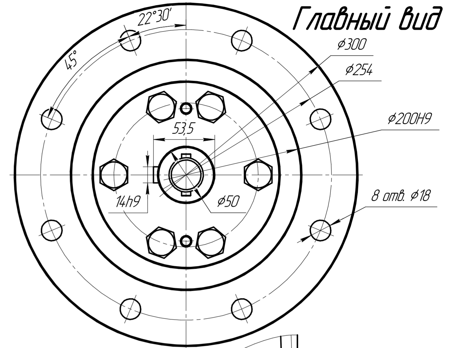
Рис. 9. Остальное см. рис. 1 F25 (B3) (15.XX) по ISO 5210 (F25M ГОСТ Р 55510)
