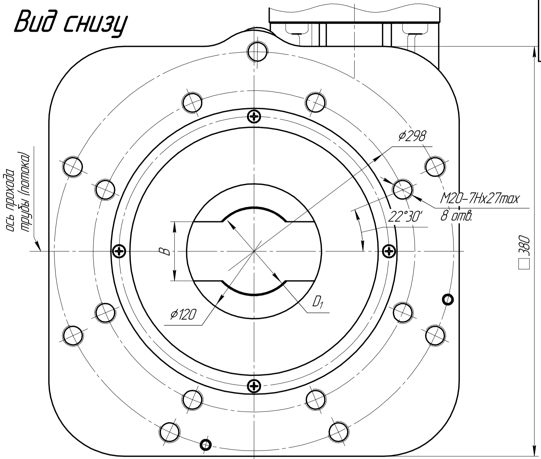
Рис. 17. Остальное см. рис. 1 на основе F30 (group C) по ISO 5210
