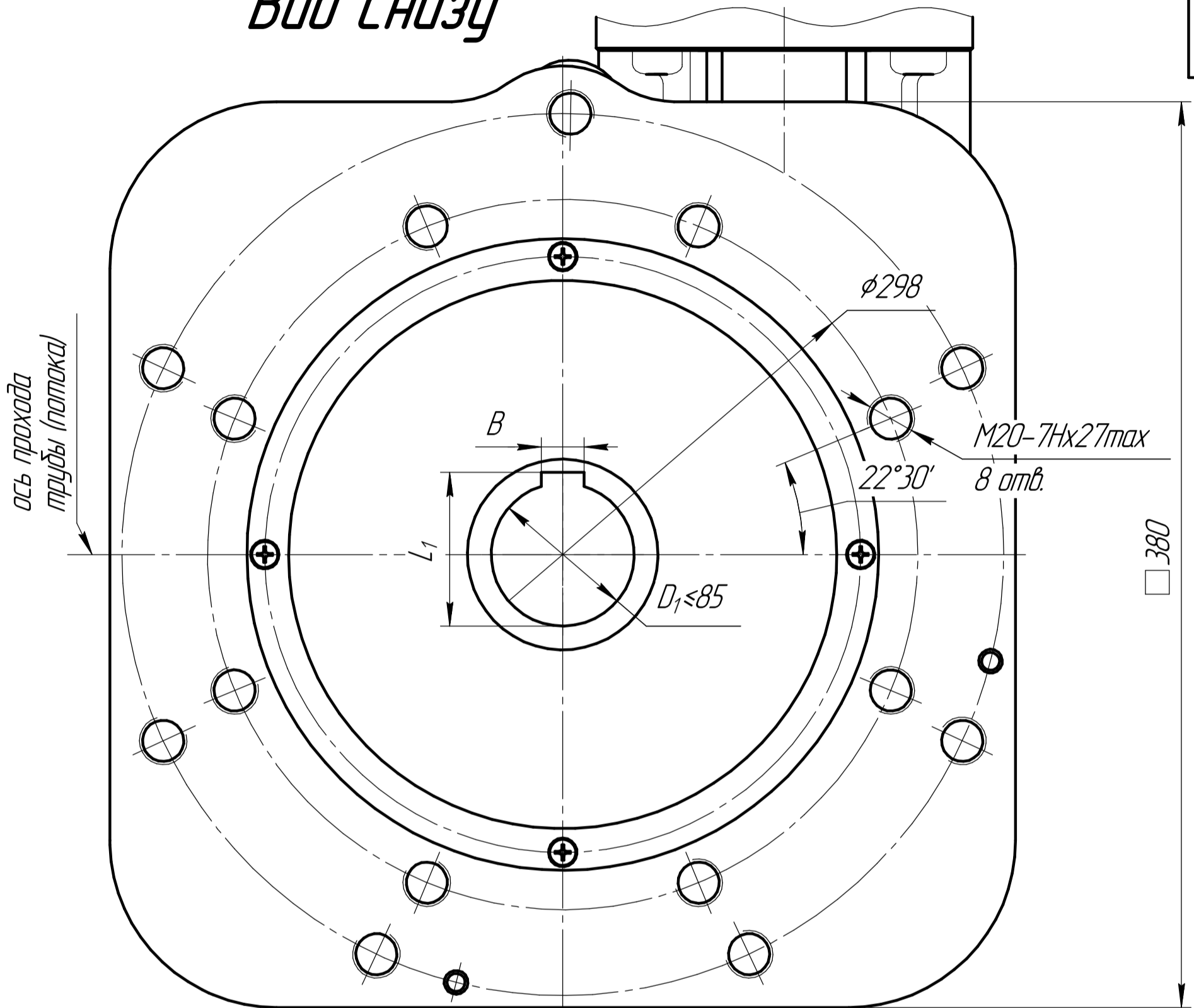
Рис. 3. Остальное см. рис. 1 F30 (Group B) по ISO 5210 (F30M (Группа B) ГОСТ Р 55510)
