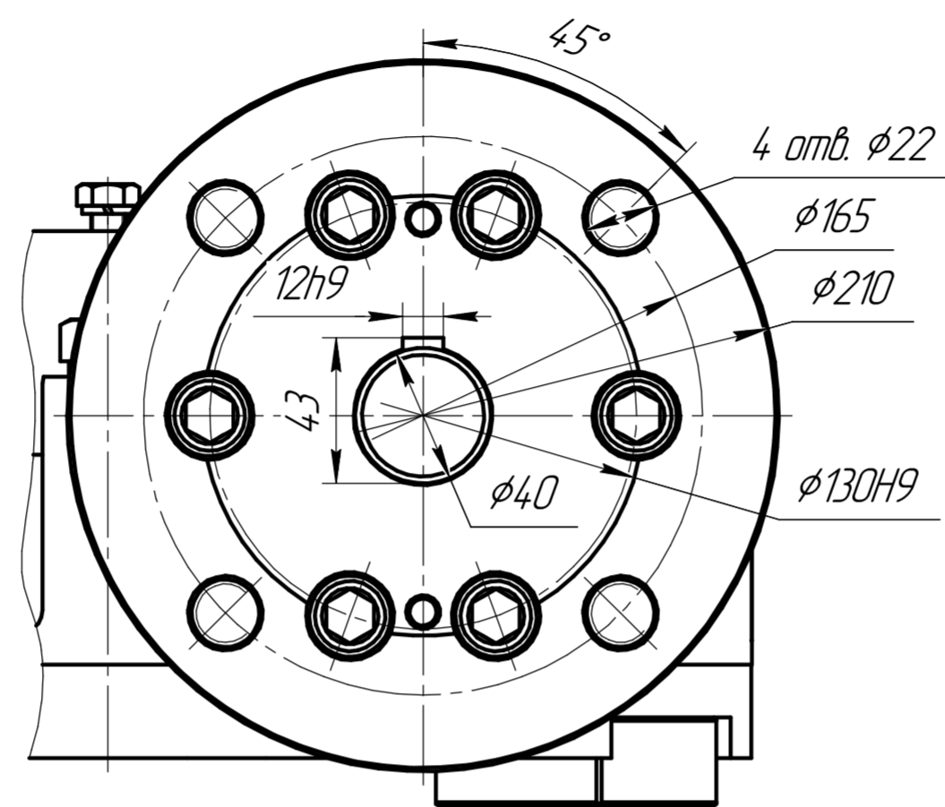
Рис. 8. Остальное см. рис. 1 F16 (B3) (14.XX) по ISO 5210 (F16M ГОСТ Р 55510) Главный вид
