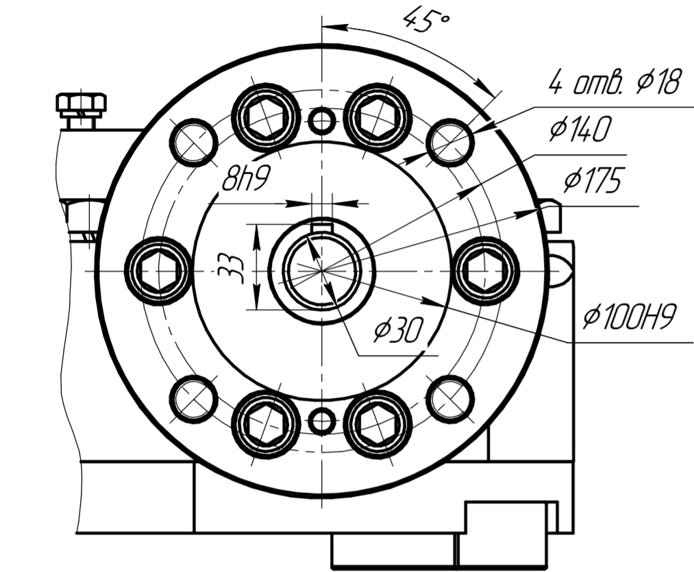
Рис. 7. Остальное см. рис. 1 F14 (B3) (13.XX) по ISO 5210 (F14M ГОСТ Р 55510) Главный вид
